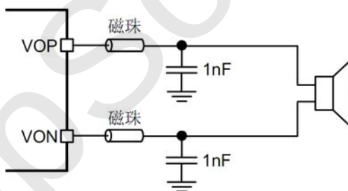
图8 磁珠与电容
